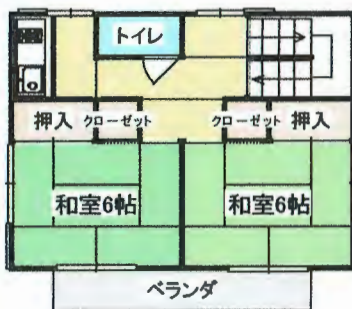
3階平面図
